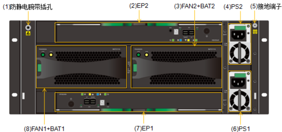
图3-19 DSU2624B 后正视图
