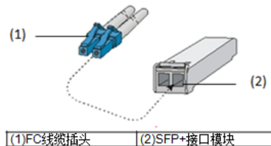
图4-36 FC 线缆和接口示意图
