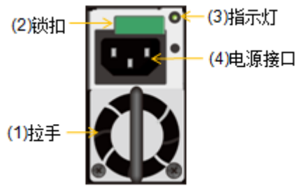
图3-25 DSU2624B/DSU2624 电源模块正视图
