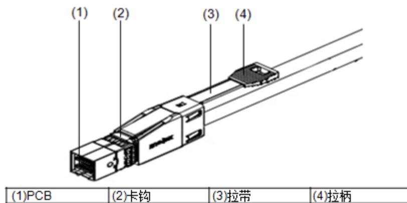
图4-31 SAS 线缆上 Mini SAS HD 连接器示意图
