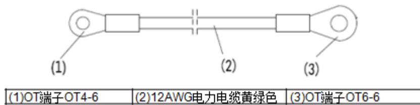
图4-23 接地线示意图
