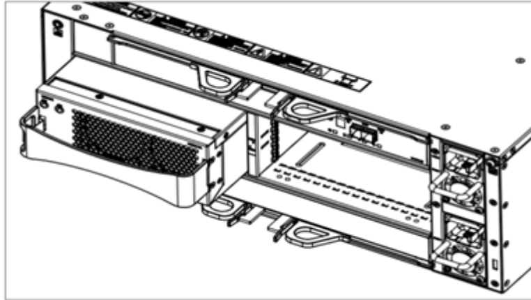
图6-9 安装/拆卸 DSU2624B 风扇模块+电池模块示意图
