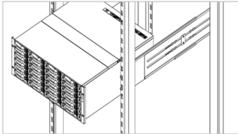
图4-17 安装 DSU 示意图
