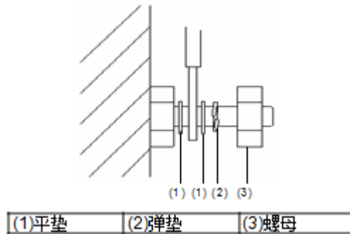
图4-18 固定线缆端子示意图
