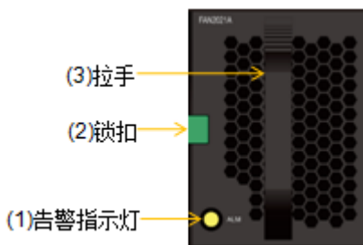
图3-15 DSU2625 风扇模块正视图
