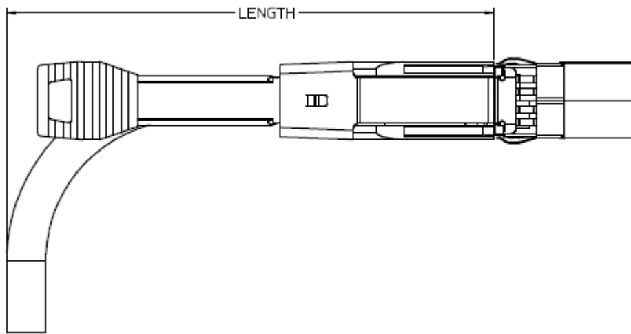
图4-32 铜缆弯曲半径示意图
