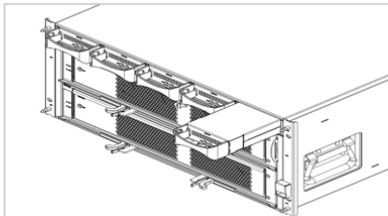
图6-4 安装/拆卸 SPU 电池模块示意图
