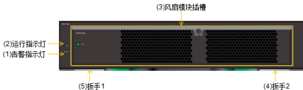
图3-4 SP 正视图
