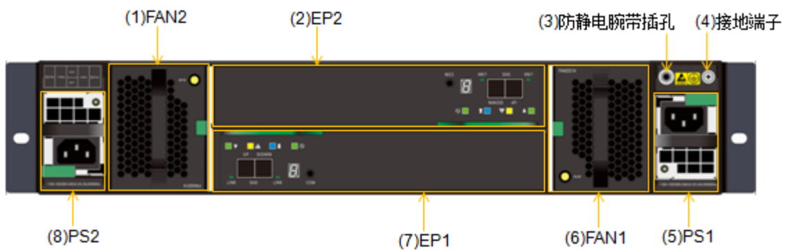
图3-11 DSU2625 后正视图
