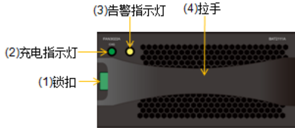
图3-23 DSU2624B 风扇模块+电池模块正视图
