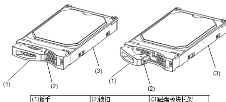
图6-17 3.5英寸磁盘模块示意图
