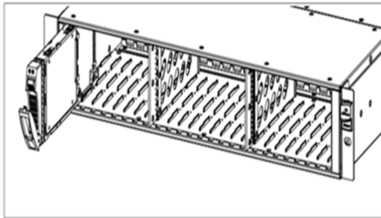
图6-16 安装 2.5 英寸磁盘模块示意图
