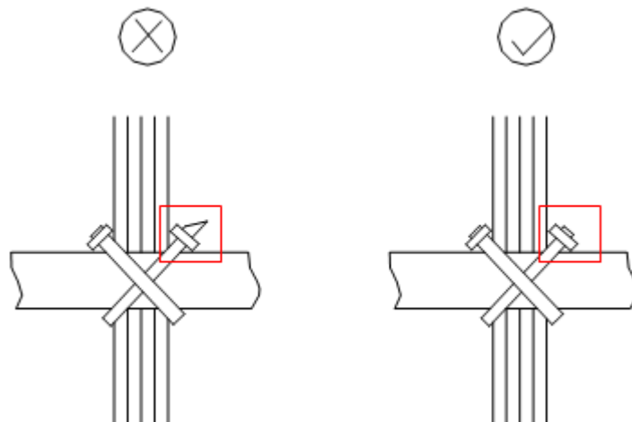
图4-20 线缆捆扎示意图（二）
