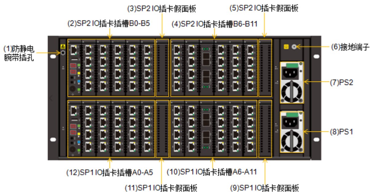
图3-3 SPU 后正视图
