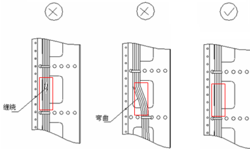
图4-19 线缆捆扎示意图（一）
