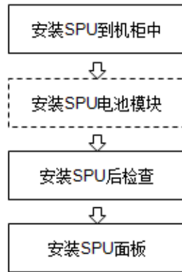
图4-12 SPU 安装流程示意图
