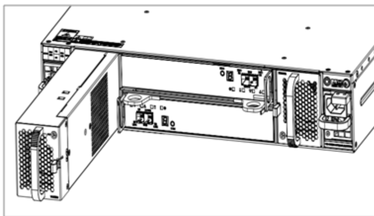
图6-10 安装/拆卸 DSU2625 风扇模块示意图
