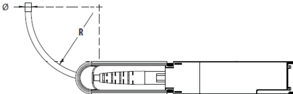
图4-33 AOC 光缆弯曲半径示意图
