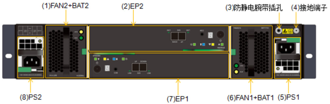
图3-10 DSU2625B 后正视图
