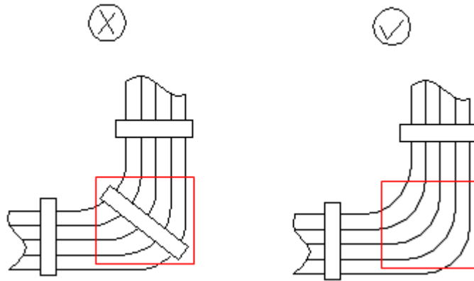
图4-21 线缆捆扎示意图（三）
