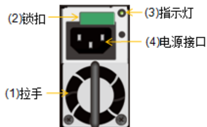
图3-8 SPU 电源模块正视图
