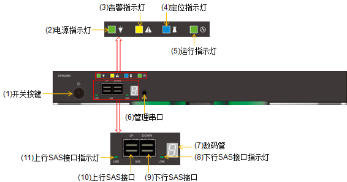
图3-21 DSU2624B 的 EP 正视图
