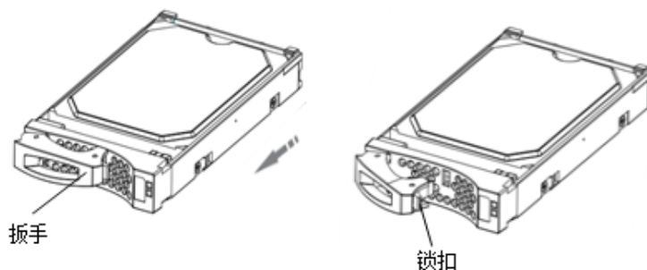
图6-19 3.5英寸磁盘模块示意图
