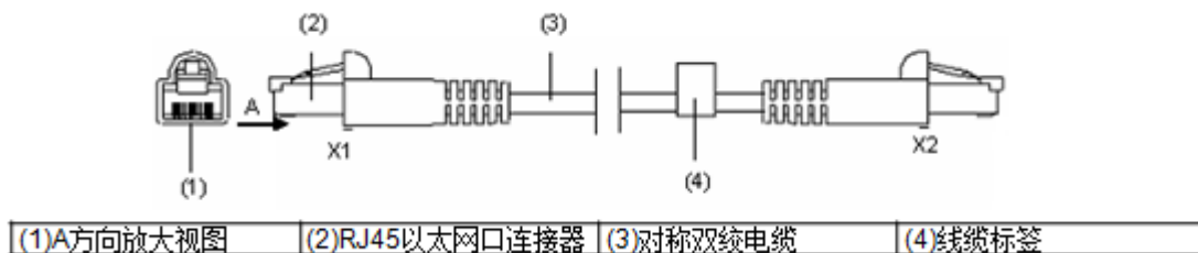
图4-37 GE 线缆示意图
