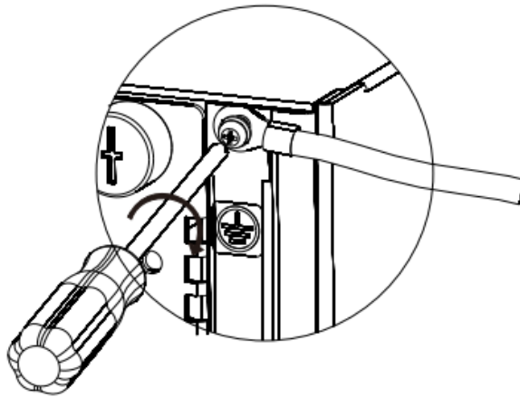
图4-25 安装接地线示意图
