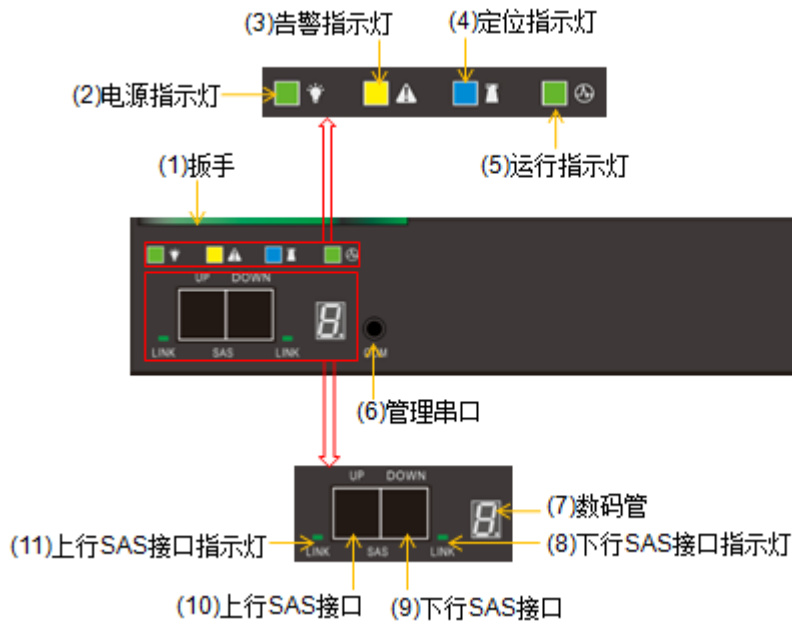
图3-13 DSU2625 的 EP 正视图
