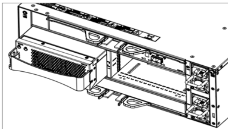
图6-11 安装/拆卸 DSU2624 风扇模块示意图
