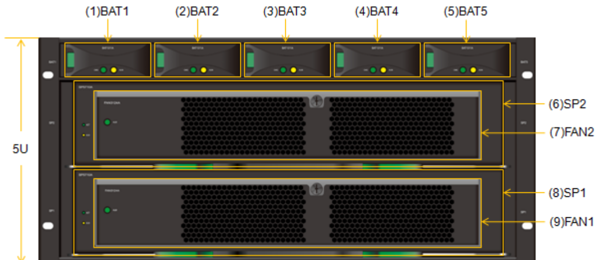
图3-2 SPU 前正视图（不带面板）
