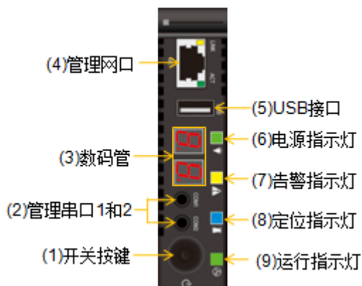
图3-5 SP 管理插卡正视图
