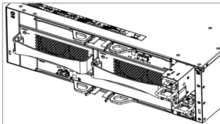
图6-12 安装/拆卸 DSU2624 电源模块示意图
