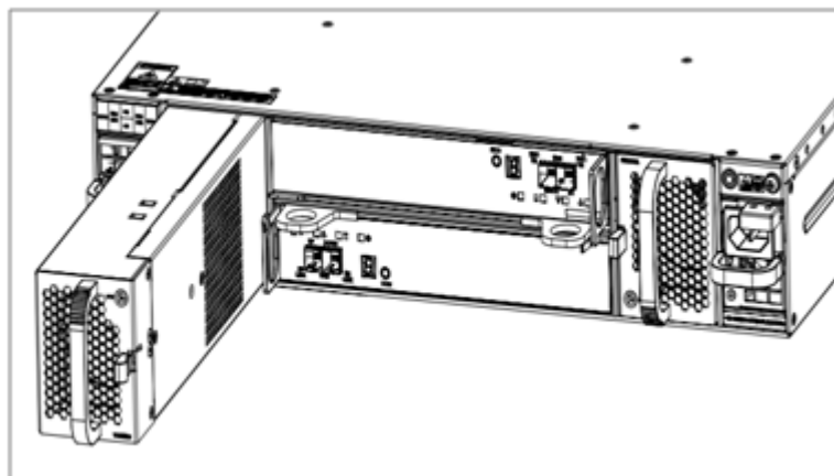
图6-8 安装/拆卸 DSU2625B 风扇模块+电池模块示意图
