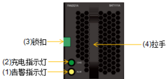
图3-14 DSU2625B 风扇模块+电池模块正视图
