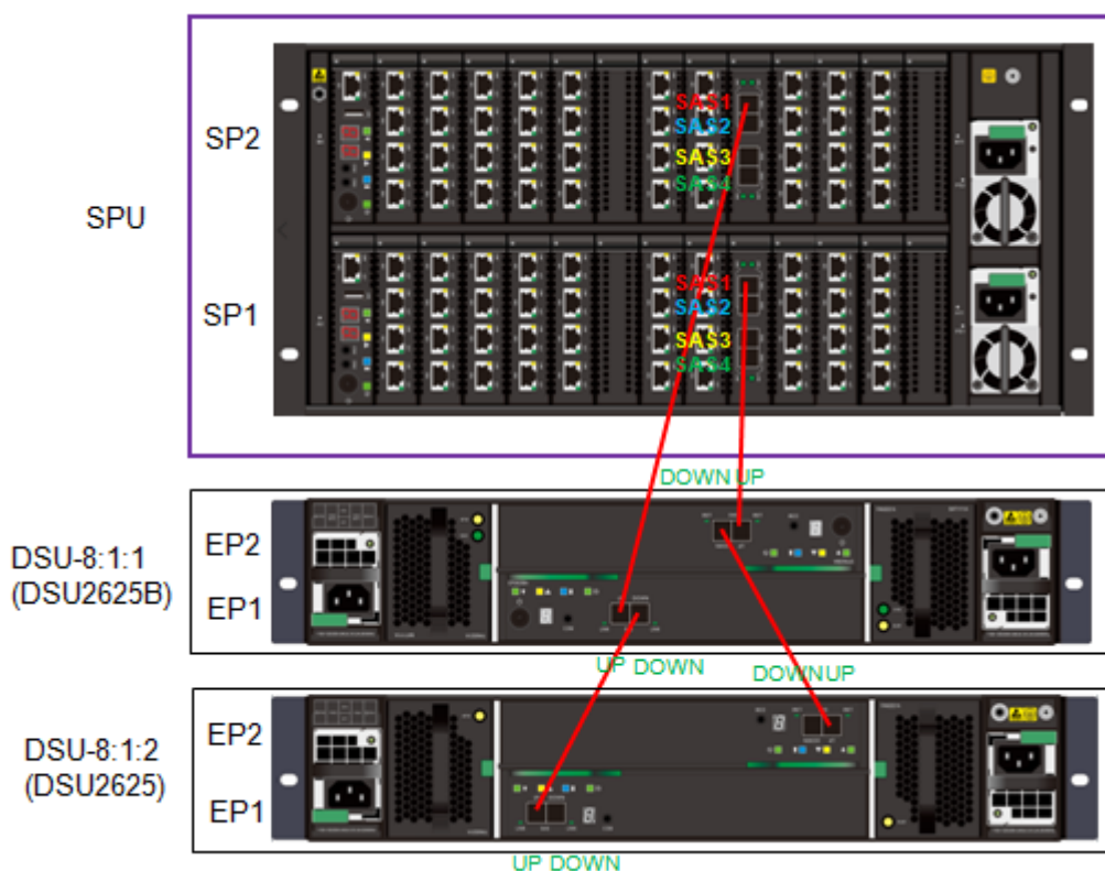
图4-34 SAS1 接口上 SAS 线缆安装示意图
