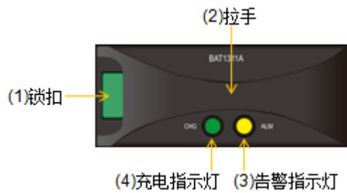
图3-7 SPU 电池模块正视图
