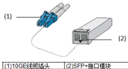
图4-38 10GE 线缆和接口示意图
