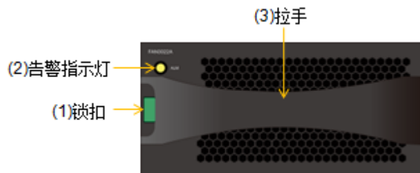
图3-24 DSU2624 风扇模块正视图
