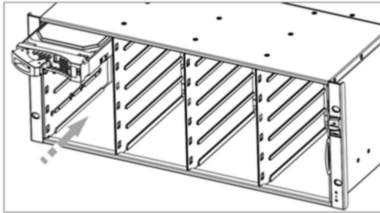
图6-20 安装 3.5 英寸磁盘模块示意图
