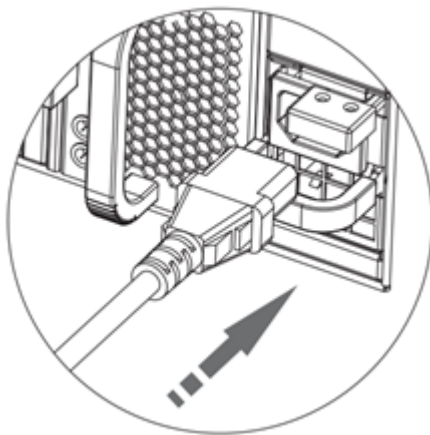
图4-28 安装电源线示意图（二）
